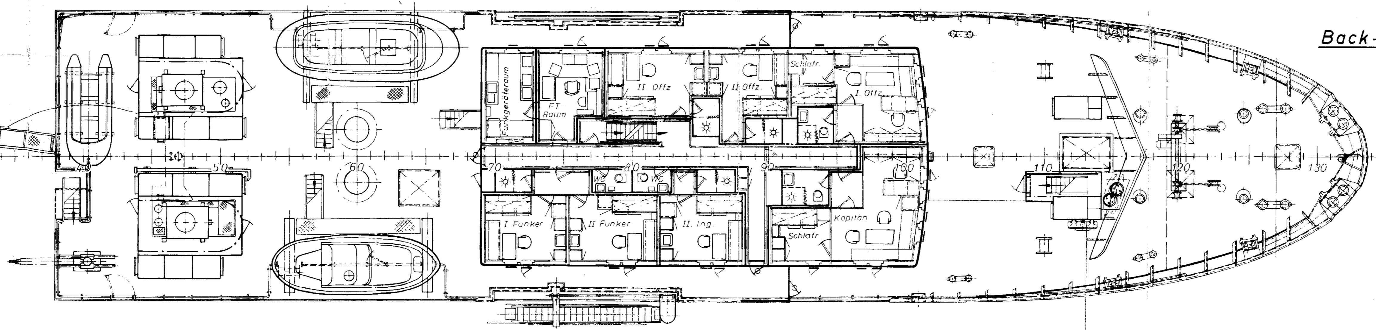
Hauptdeck
